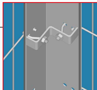
Fixador Gaivota®
